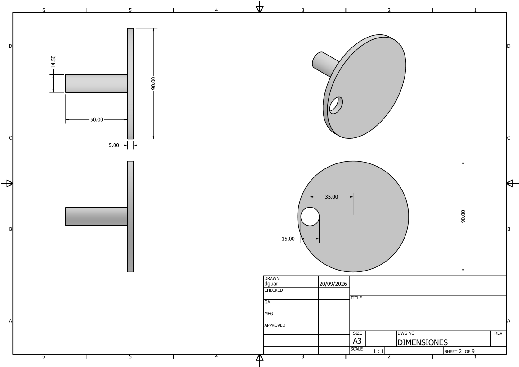
Figura 19. Hoja 2: Disco-manivela (escala 1:1).
