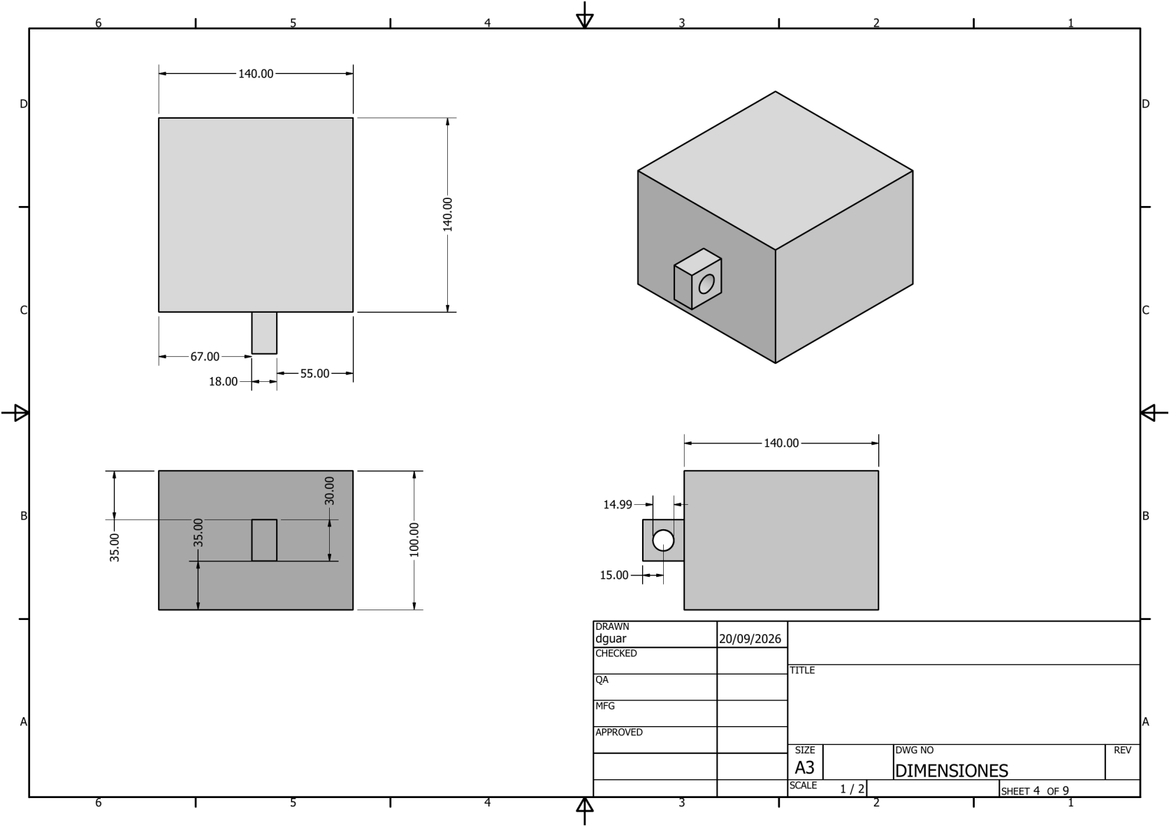
Figura 21. Hoja 4: Bloque (pisón) (escala 1:2).
