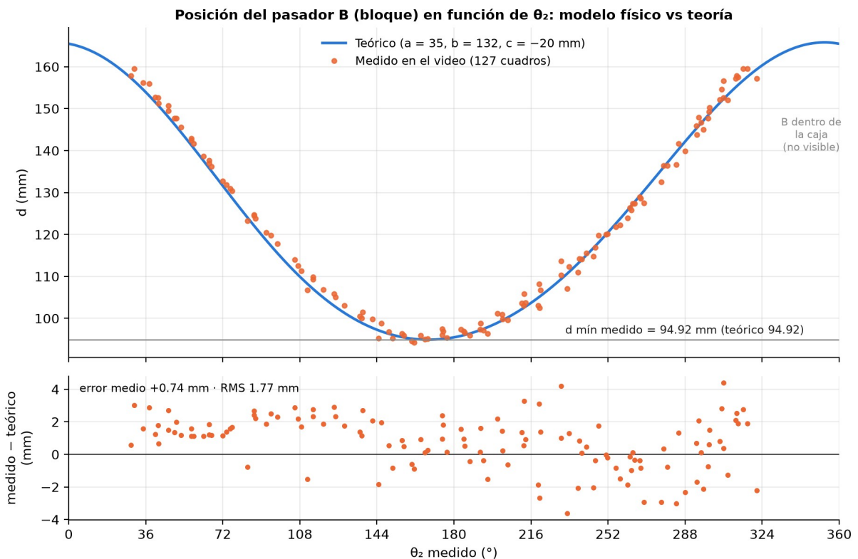
Figura 12. Posición del pasador B del bloque medida en el video contra la curva teórica, en función del ángulo medido de la manivela. Abajo: diferencia medido – teórico.
