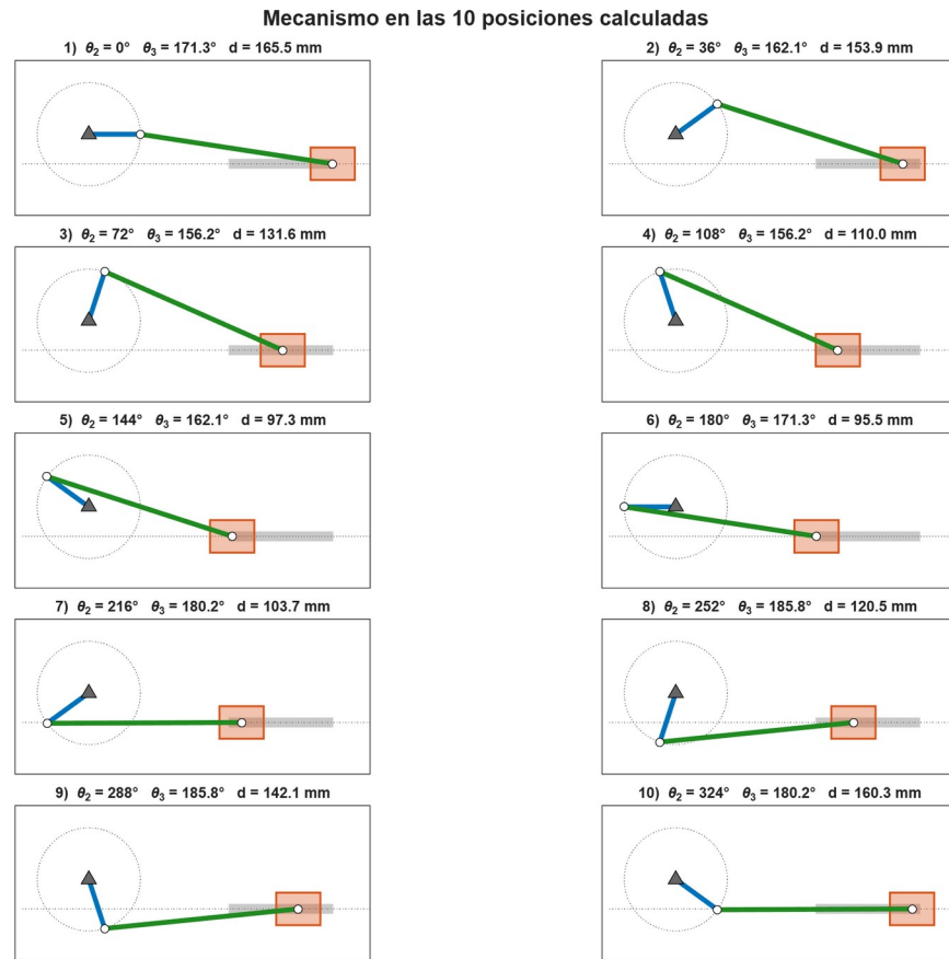
Figura 7. El mecanismo en las 10 posiciones calculadas (MATLAB). La franja gris es la carrera del bloque.
