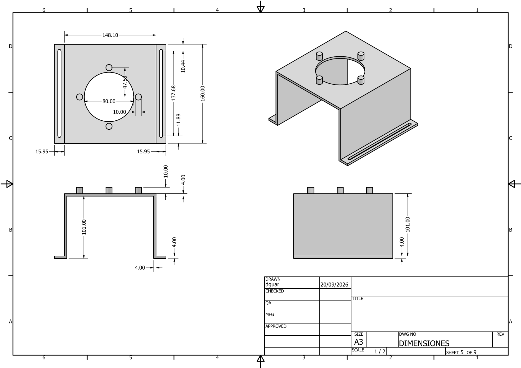
Figura 22. Hoja 5: Caja-guía (escala 1:2).
