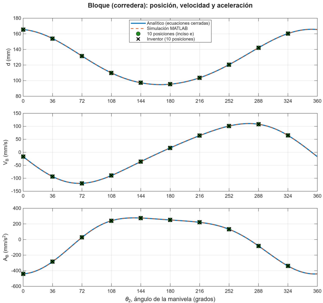
Figura 9. Posición, velocidad y aceleración del bloque (eslabón de salida) contra \theta_2 .
