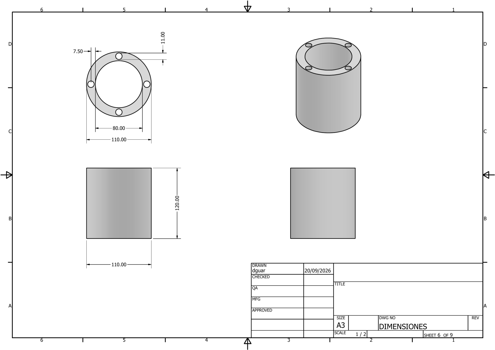
Figura 23. Hoja 6: Tolva (escala 1:2).
