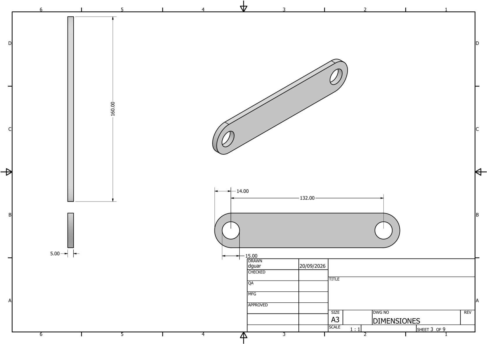
Figura 20. Hoja 3: Biela (escala 1:1).
