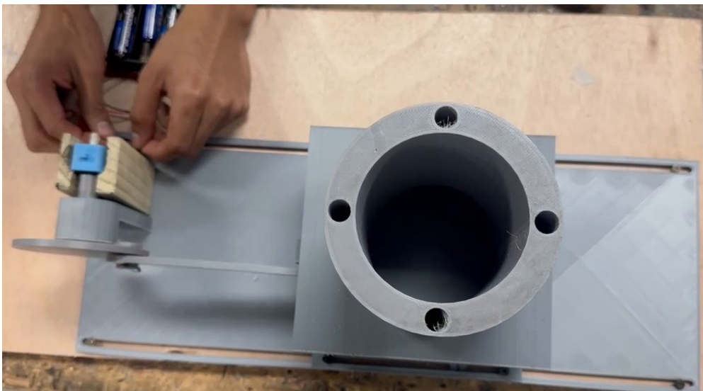
Figura 5. Vista superior del modelo físico: motor sujeto en el soporte de madera junto al disco-manivela, biela, caja-guía y tolva.
