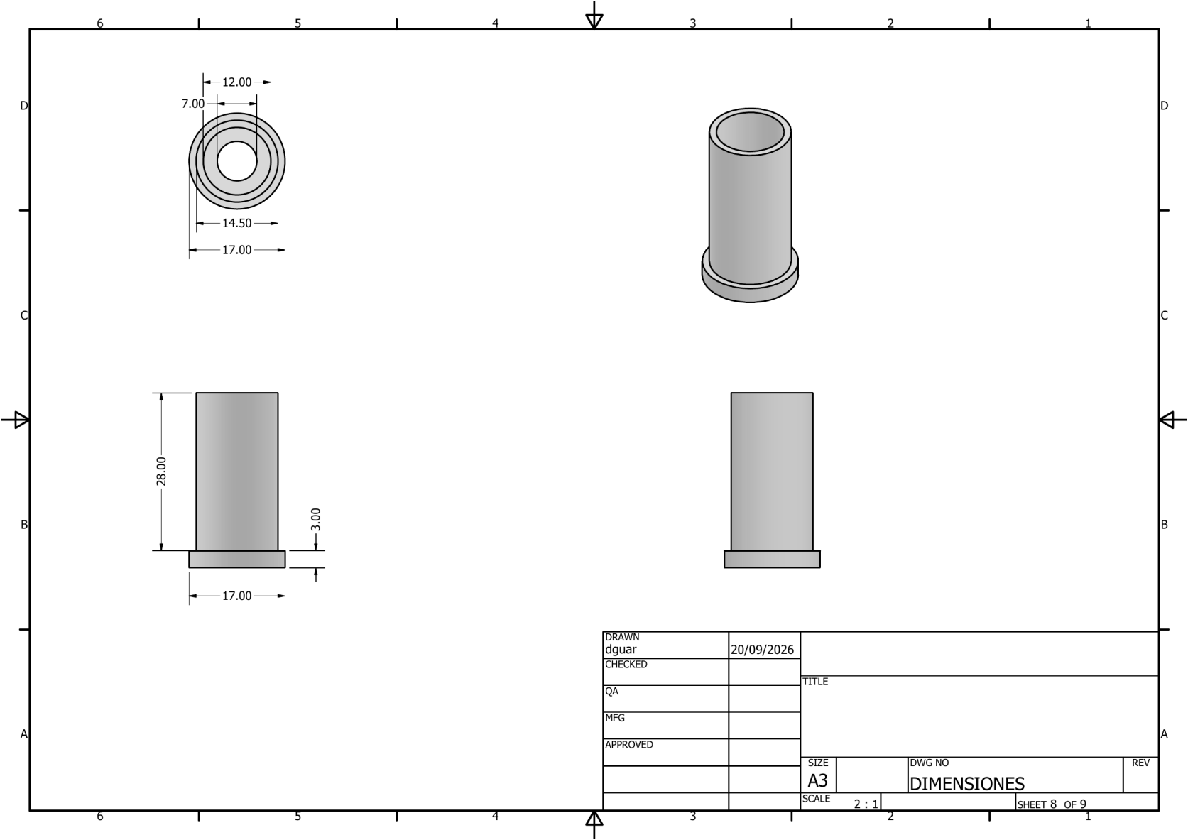
Figura 24. Hoja 8: Pasador-buje (escala 2:1).
