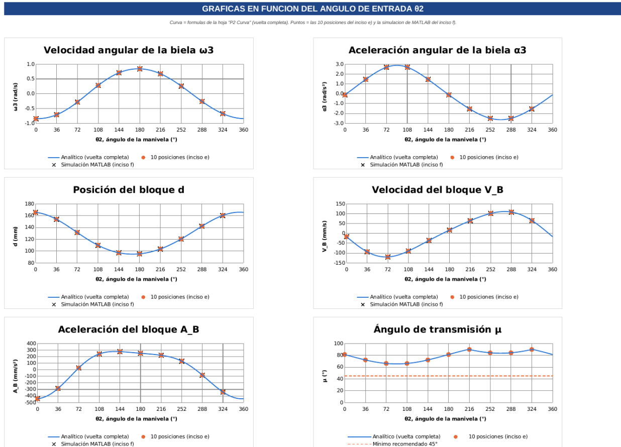
Figura 17. Hoja "P2 Graficas" del Excel: variables del mecanismo en función del ángulo de entrada.
