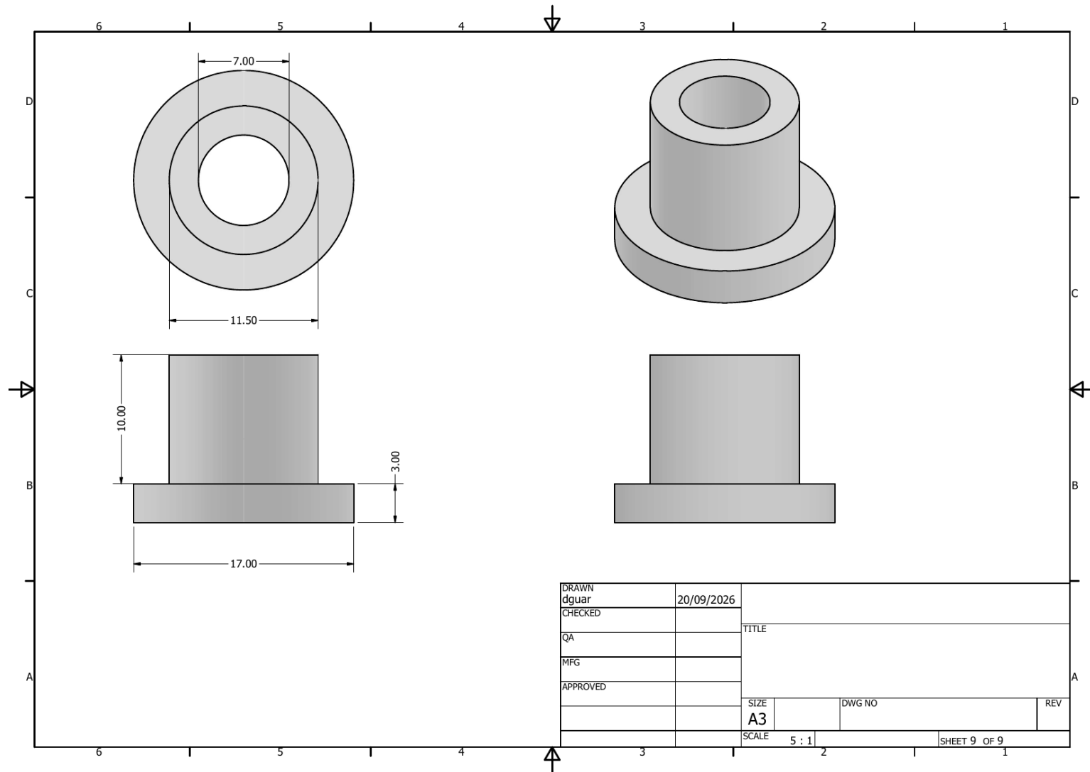
Figura 25. Hoja 9: Tapa del pasador (escala 5:1).
