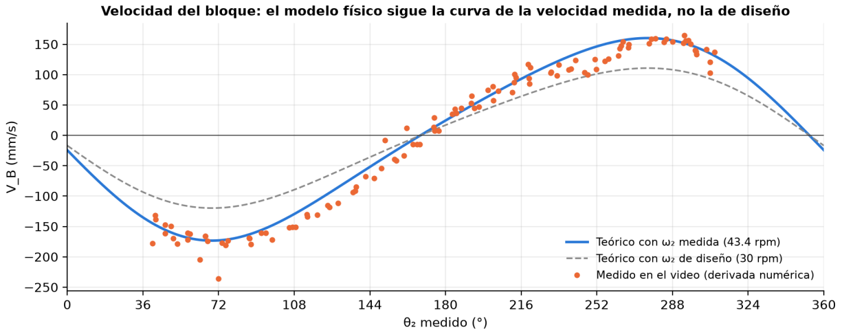
Figura 13. Velocidad del bloque medida (derivada numérica de la posición) contra la teórica con la velocidad medida del motor y con la de diseño.
