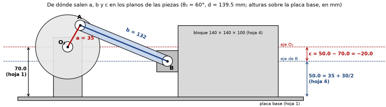
Figura 3. Cómo salen a , b y c de los planos: alturas del eje O_2 (soporte, hoja 1) y del pasador B (oreja del bloque, hoja 4) sobre la placa base. Dibujo a escala con \theta_2 = 60^\circ .
