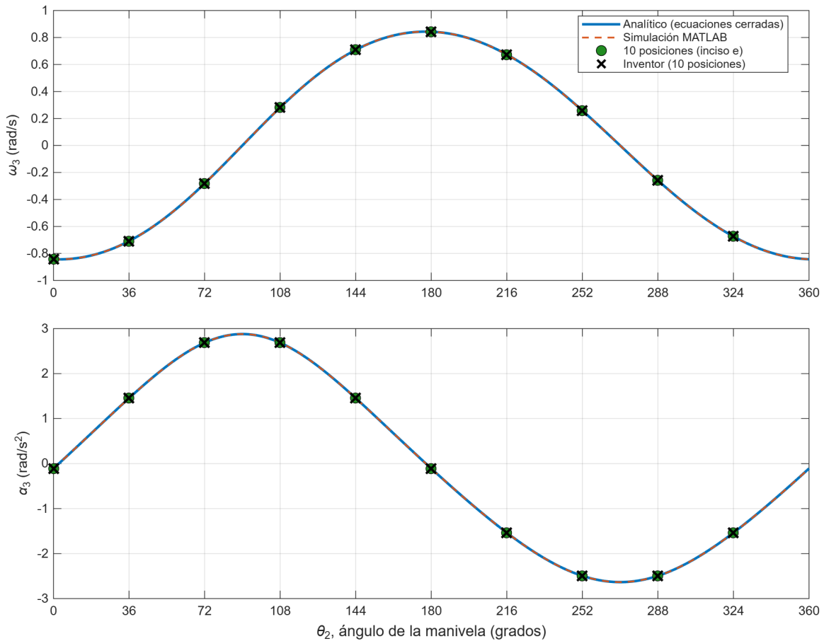
Figura 8. Velocidad y aceleración angular de la biela contra \theta_2 : ecuaciones cerradas (línea), simulación en MATLAB (línea discontinua), 10 posiciones del inciso e (círculos) e Inventor (cruces).
