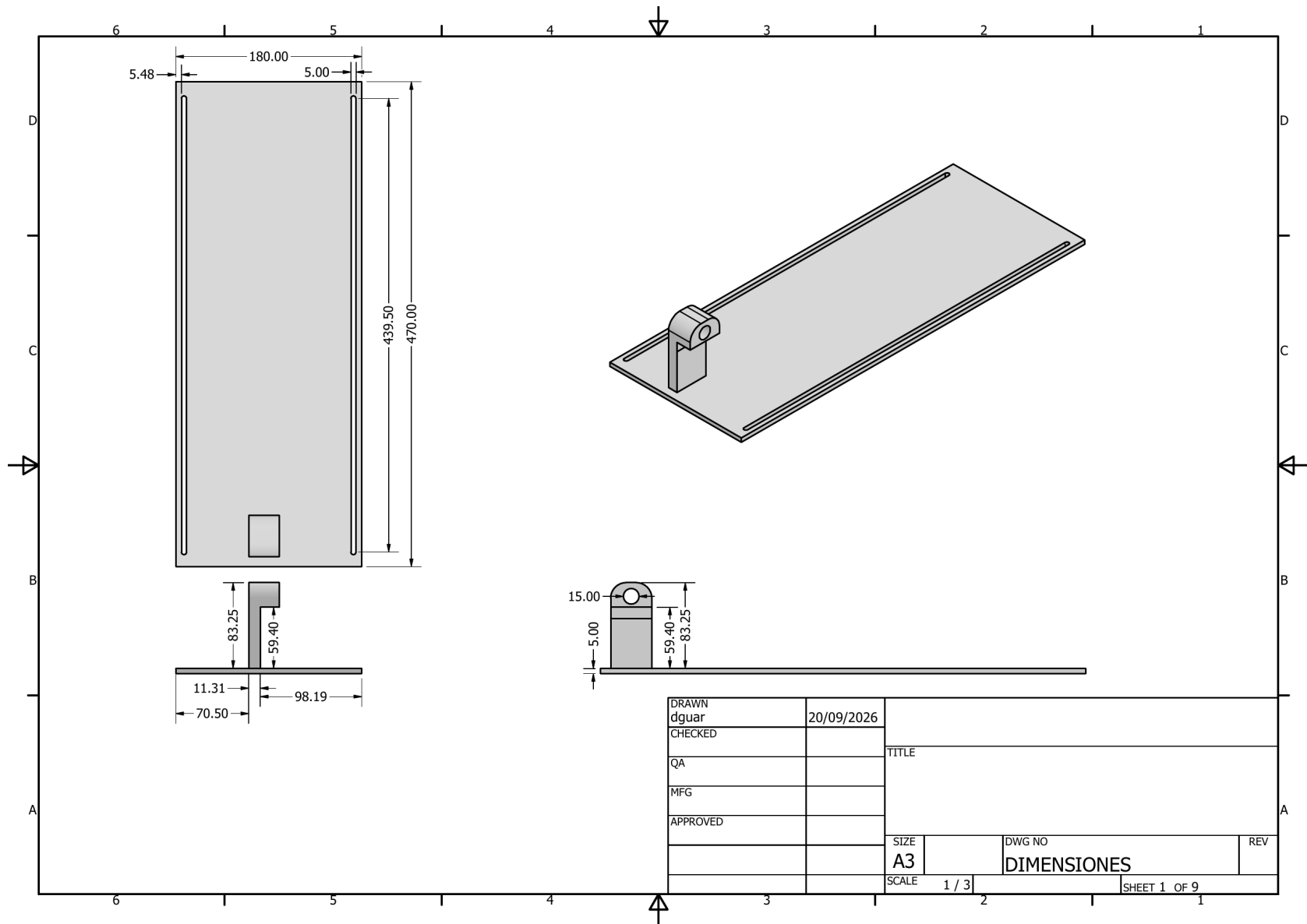
Figura 18. Hoja 1: Base con soporte de la manivela (escala 1:3).
